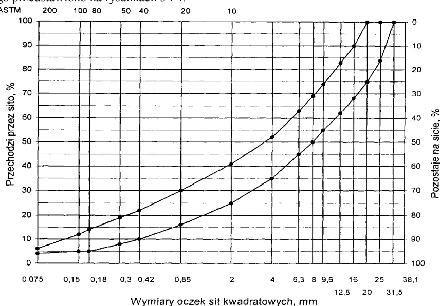
Rys. 3. Krzywe graniczne uziarnienia mieszanki mineralnej BA od 0 do 20 mm do warstwy wiążącej, wyrównawczej i wzmacniającej nawierzchni drogi o obciążeniu ruchem od KR3 do KR6
